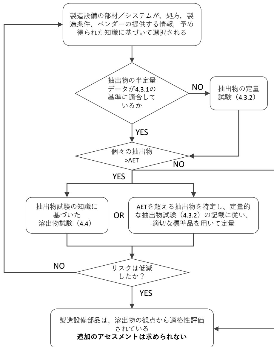
図4：製造の部材／システムに関連するE&L評価におけるリスクの特定及び低減に関する典型的なワークフロー
